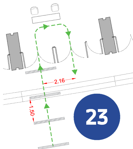
Imatge 6. Muntatge tipus de l'accés 23, sentit d'entrada i de sortida i marques al paviment indicant distància de 1,50m.
